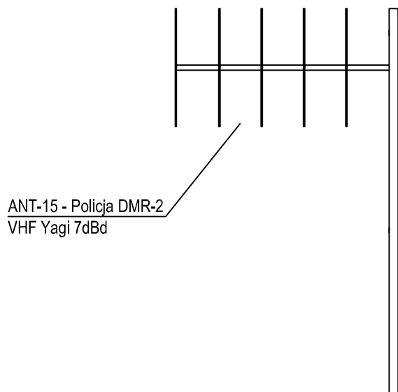
MASZT ANTENOWY 8 h=3m
