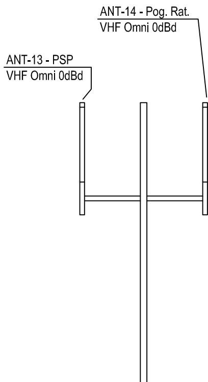
MASZT ANTENOWY 7 h=3m
