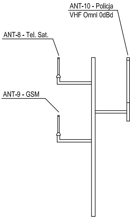
MASZT ANTENOWY 5 h=3m
